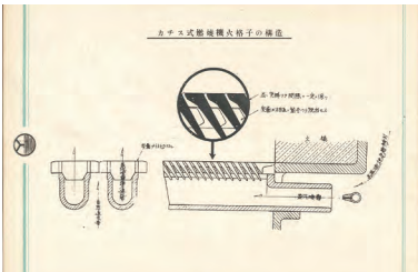
カチス式粗悪炭完全燃焼機器カタログ(吉嶺工業所)
