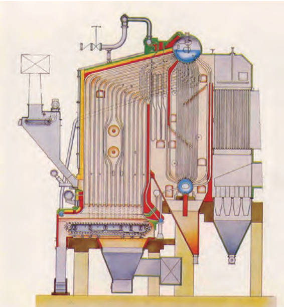
H型ボイラ (よしみねトラベリングストーカー 1号機: 昭和51年)
